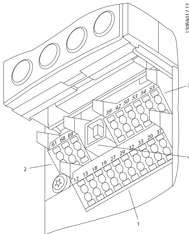
Bild 2.19 Styrplintplatser
