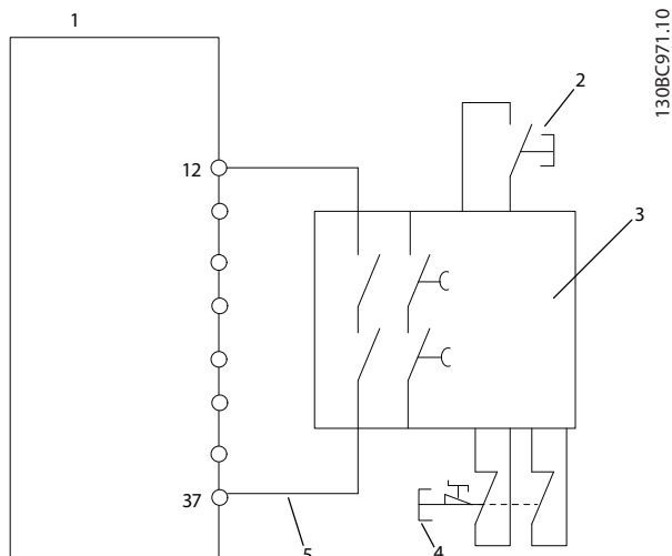
Bild 2.28 Installation för att uppfylla stoppkategori 0 (SS-EN 60204-1) med kat. 3/PL "d" (ISO 13849-1) eller SIL 2 (SS-EN 62061).
