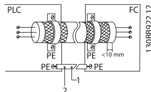
Bild 2.22 Korrekt skärmning
