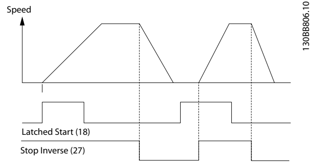
Bild 6.2 Pulsstart/stopp, inverterat
