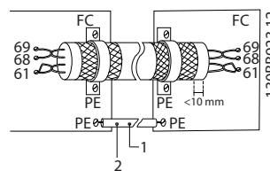
Bild 2.24 Tvistade kablar
