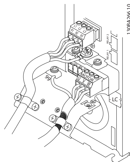
図 2.7 シールド・ケーブルによる接地
