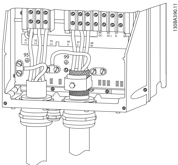
図 2.9 B、C および D フレームサイズでシールド・ケーブルを使用した場合のモーター、主電源、アース配線
