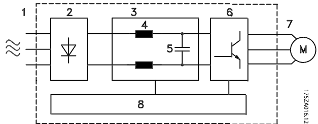
図 1.3 周波数変換器ブロック図
