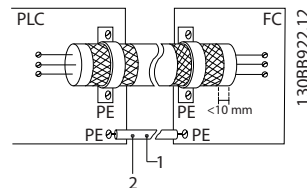
Ilustracja 2.22 Prawidłowe ekranowanie
