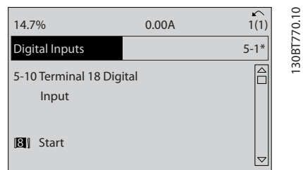
Ilustracja 5.11 Wejścia cyfrowe
