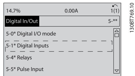
Ilustracja 5.10 Wej./Wyj.cyfr.
