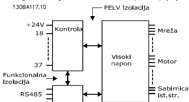
Slika 8.1 PELV izolacija
