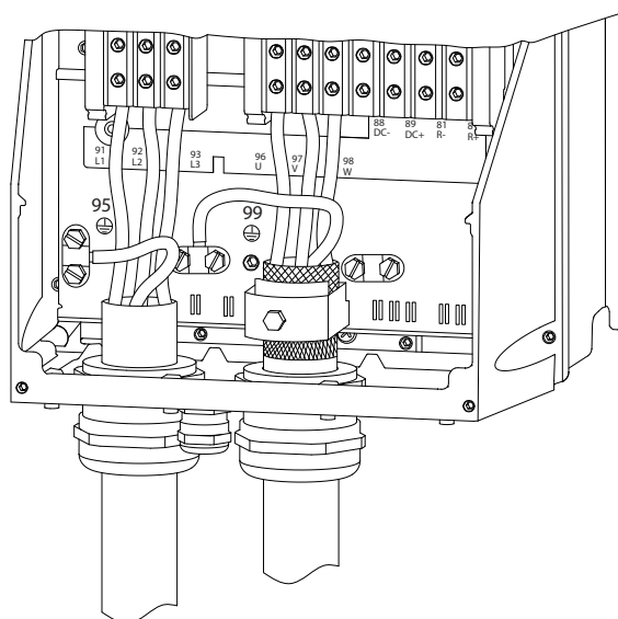
Slika 4.8 Motor, mrežno napajanje i ožičenje uzemljenja za tipove kućišta B i C sa kablom sa omotačem
