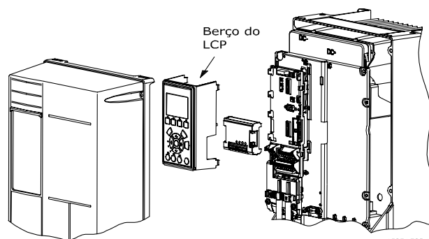
Ilustração 3.2 Tipos de gabinetes A5, B1, B2, B4, C1, C2, C3 e C4
