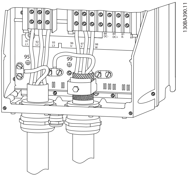
Ilustração 6.18 Conexão do motor para gabinete metálico tipo C1 e C2 (IP21/NEMA tipo 1 e IP55/66/NEMA tipo 12)
