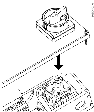
Ilustração 6.39 Localização do interruptor de rede elétrica
