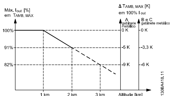
Ilustração 9.24 Derating da corrente de saída versus altitude a T_{AMB, MÁX.} para gabinetes metálicos tipos A, B e C. Em altitudes superiores a 2.000 m, entre em contato com a Danfoss em relação à PELV
