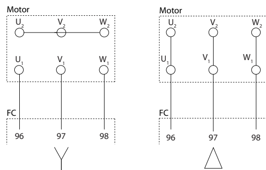
Ilustração 6.20 Conexões delta e em estrela
