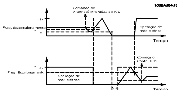
Ilustração 7.8 Escalonamento de Bomba com Alternação da Bomba de Comando
