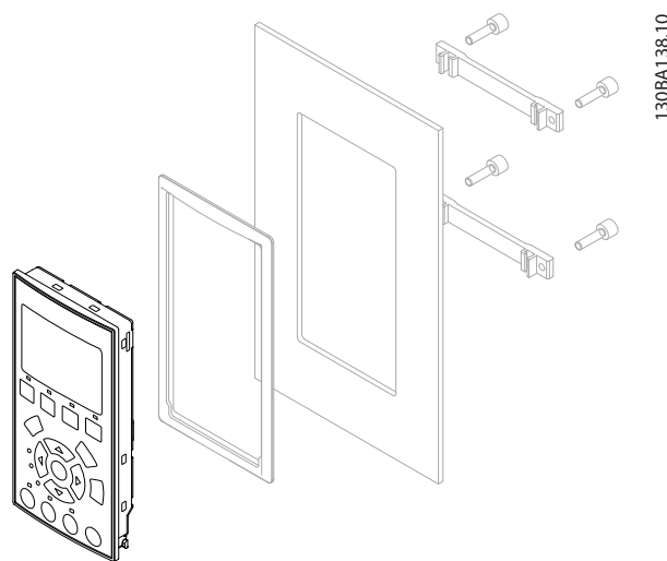
Ilustração 3.16 Kit de LCP com LCP Gráfico, Presilhas, Cabo de 3 m e Guarnição Nº de Pedido 130B1113
