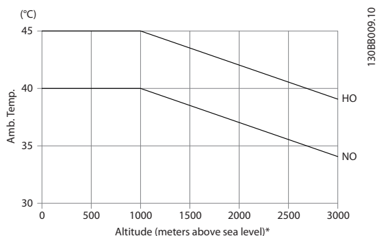
Ilustração 9.26 Exemplo: A uma altitude de 2.000 m e uma temperatura de 45 °C ( T_{AMB, MÁX.} - 3,3 K), 91% da corrente de saída nominal está disponível. Na temperatura de 41,7 °C, 100% da corrente de saída nominal fica disponível
