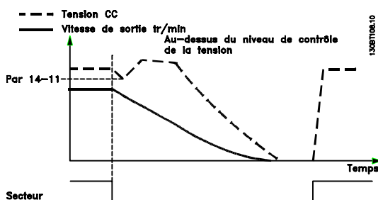
Illustration 3.35 Rampe de décélération contrôlée, défaut secteur plus long. Décélération tant que l'énergie du système le permet, puis mise en roue libre du moteur.
