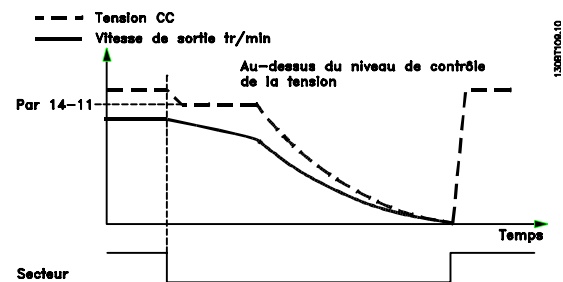
Illustration 3.37 Sauvegarde cinétique - Panne secteur plus longue. Le moteur est en roue libre dès que l'énergie du système est trop basse.
