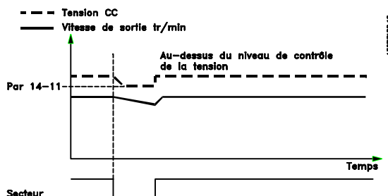
Illustration 3.36 Sauvegarde cinétique - Brève panne de secteur. Fonctionnement tant que l'énergie du système le permet.
