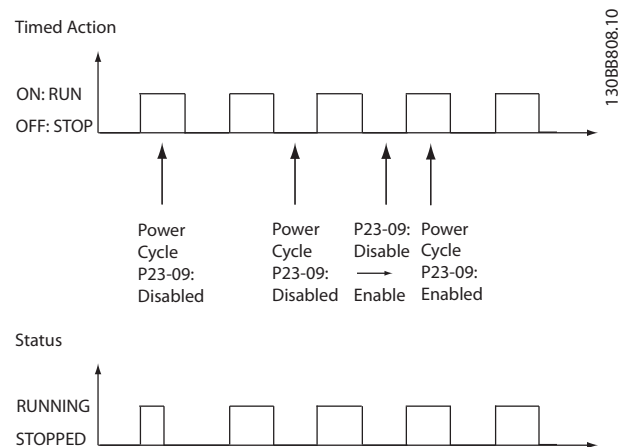
Illustration 3.59 Schéma de test de réactivation
