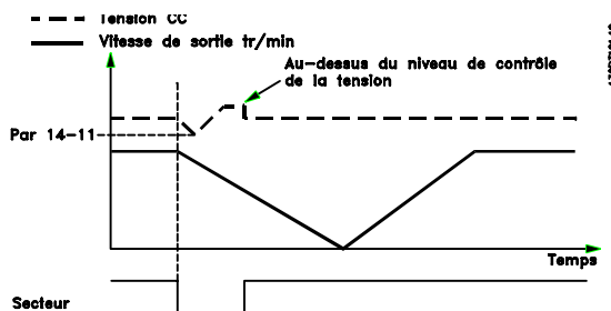
Illustration 3.34 Rampe de décélération contrôlée - Bref défaut secteur. Décélération jusqu'à l'arrêt, puis accélération jusqu'à la référence.
