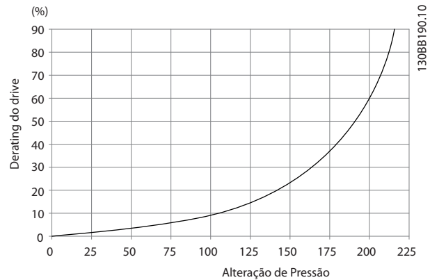
Ilustração 9.7 Derating x Mudança de pressão para gabinetes F1-F4. Fluxo de ar: 580 cfm (985 m 3 /h)
