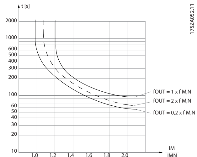
Ilustração 5.1 Características do ETR
