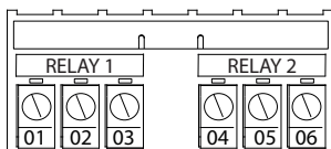
Ilustração 10.13 Terminais dos relés 1 e 2
