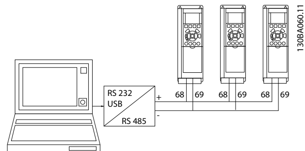
Ilustração 14.2 Conexões paralelas
