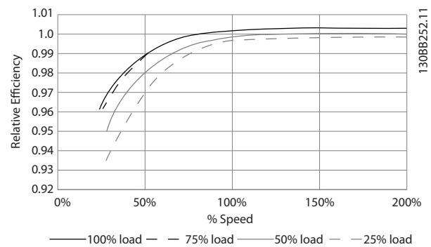
Ilustração 10.25 Curvas de eficiência típica
