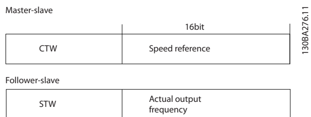
Ilustração 14.18 Valor de referência da velocidade do barramento
