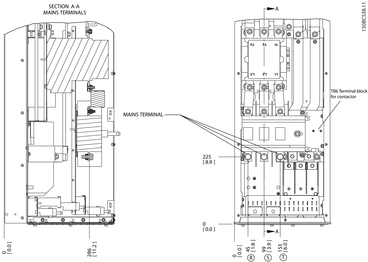
Illustration 2.16 Klemmeplaceringer, D6h med kontaktor og afbryderoptioner
