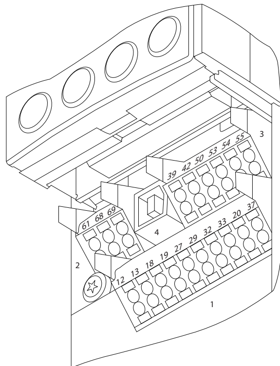
Illustration 2.29 Styreklemmeplaceringer
