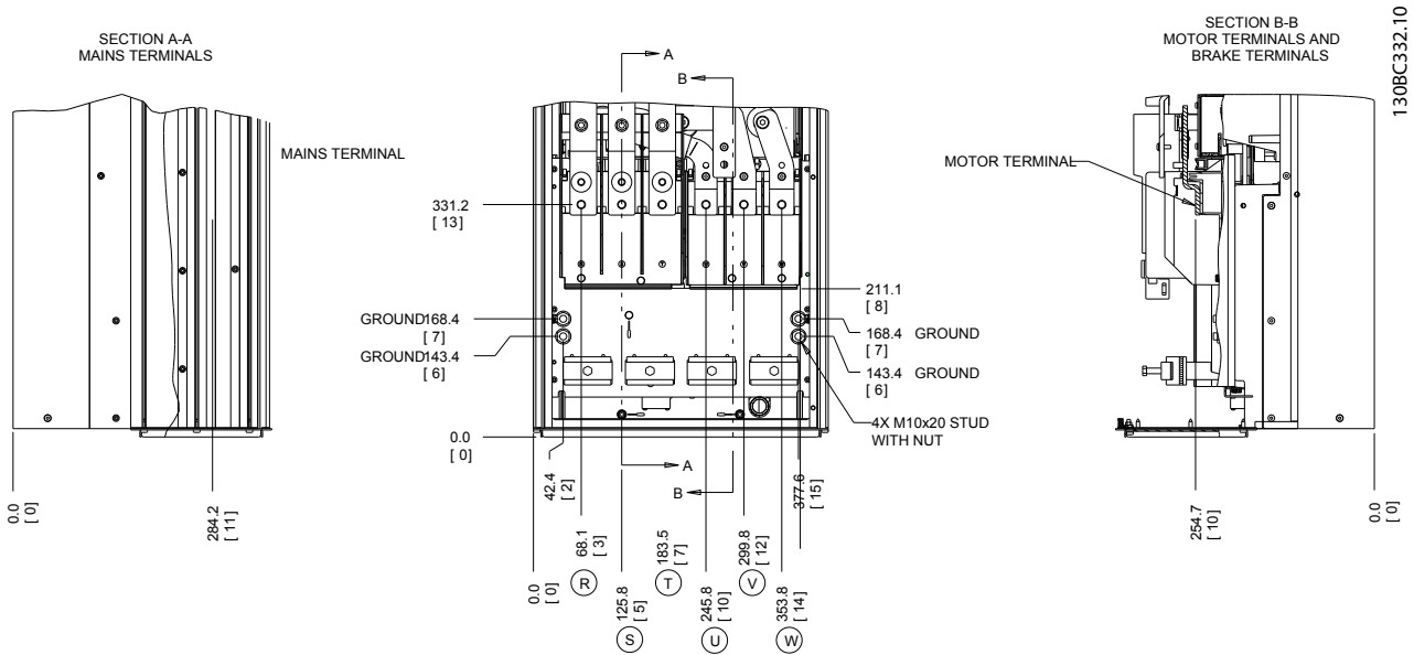
Illustration 2.10 Klemmeplaceringer D2h
