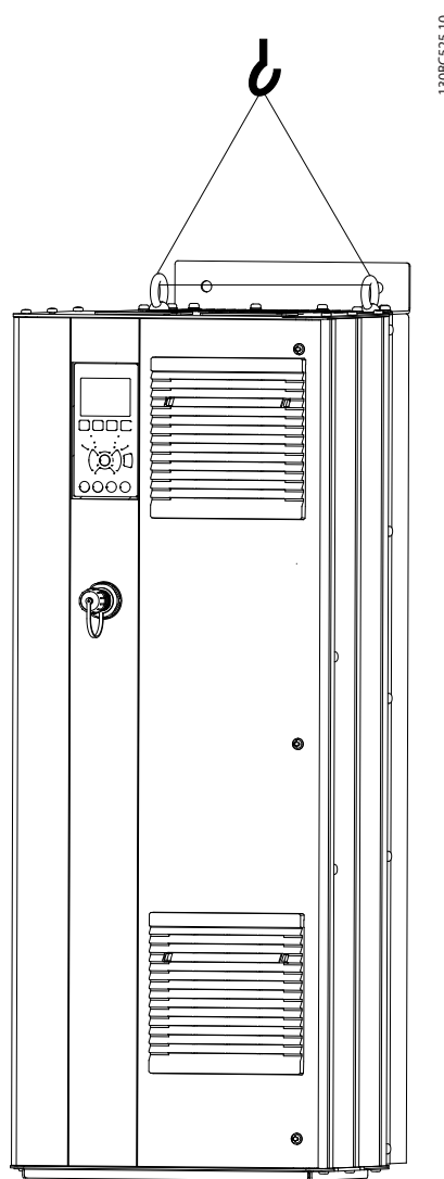
Abbildung 2.1 Empfohlenes Hebeverfahren
