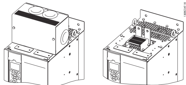
Abbildung 2.32 Zwischenkreiskopplungs- oder Regen-Klemme mit Abdeckung (L) und ohne Abdeckung (R)
