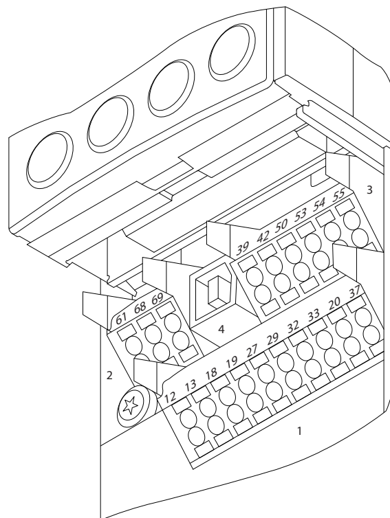
Bild 2.29 Styrplintplatser
