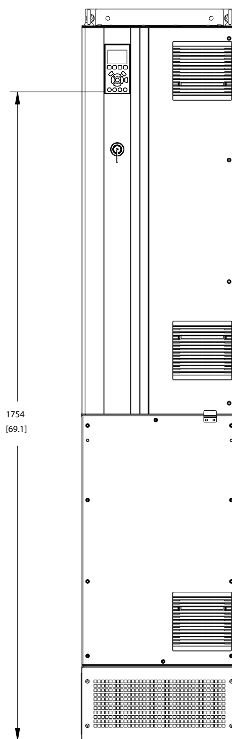
Bild 1.3 D7h-kapsling
