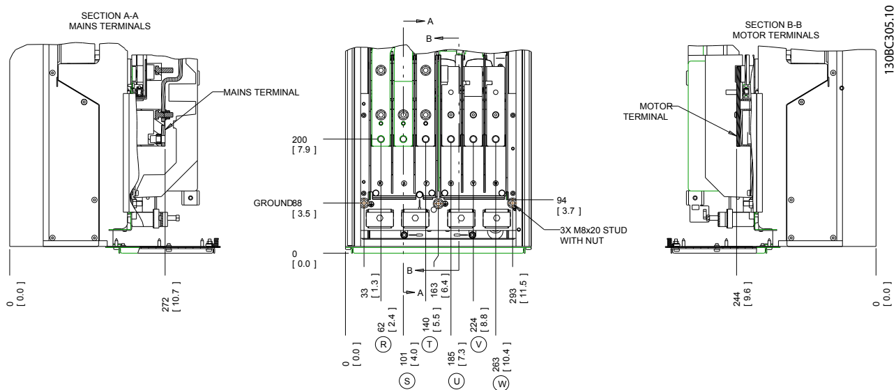
Bild 2.7 Plintplaceringar D1h
