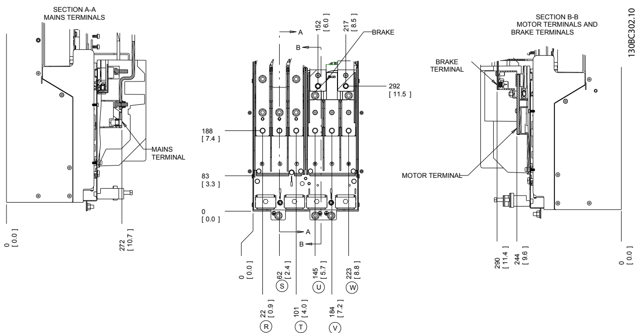
Bild 2.8 Plintplaceringar D3h
