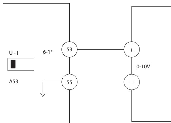
Bild 5.10 Kabeldragnings exempel för extern enhet med 0-10 V styrsignal
