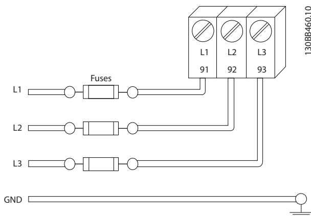
Afbeelding 2.4 Zekeringen frequentieomvormer
