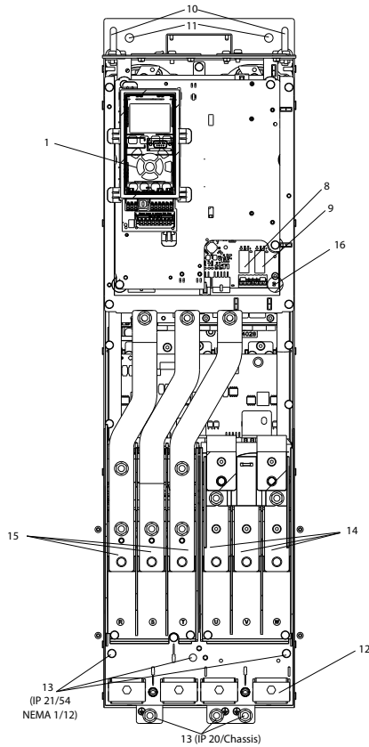
Εικόνα 1.1 D1 Εσωτερικά εξαρτήματα
