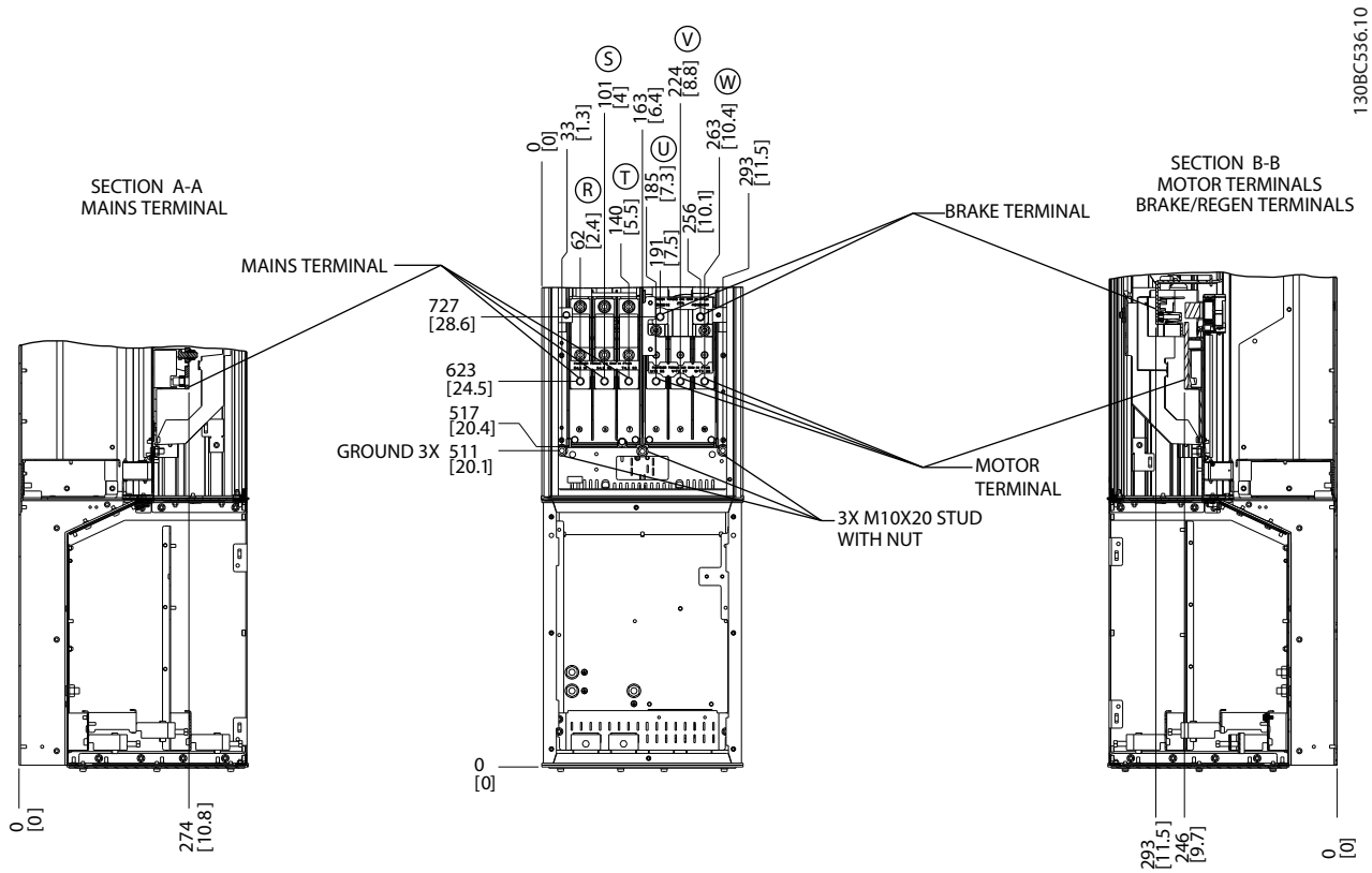
Εικόνα 2.14 Θέσεις ακροδεκτών , D5h με επιλογή πέδησης
