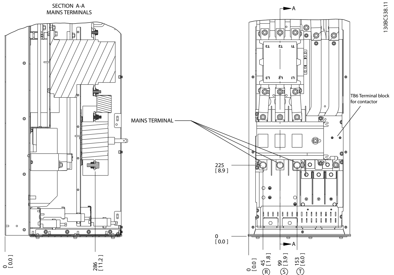
Εικόνα 2.16 Θέσεις ακροδεκτών, D6h με επιλογές Επαφές και Αποζεύκτη
