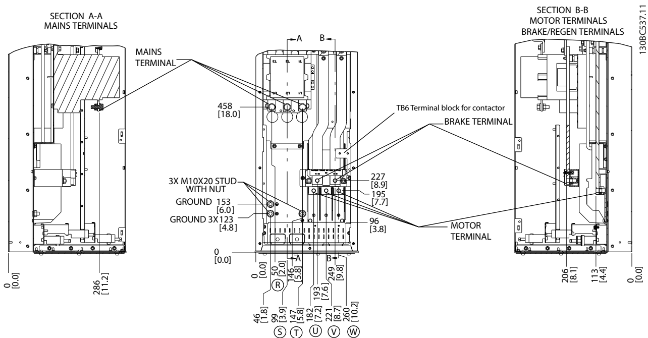
Εικόνα 2.15 Θέσεις ακροδεκτών, D6h με επιλογή Επαφά
