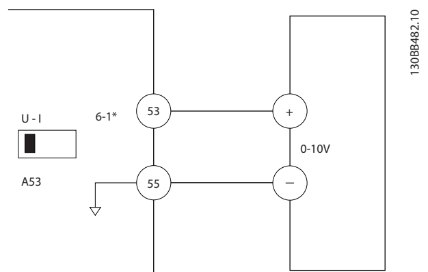
Εικόνα 5.10 Παράδειγμα καλωδίωσης για εξωτερική συσκευή που παρέχει σήμα ελέγχου 0-10 V
