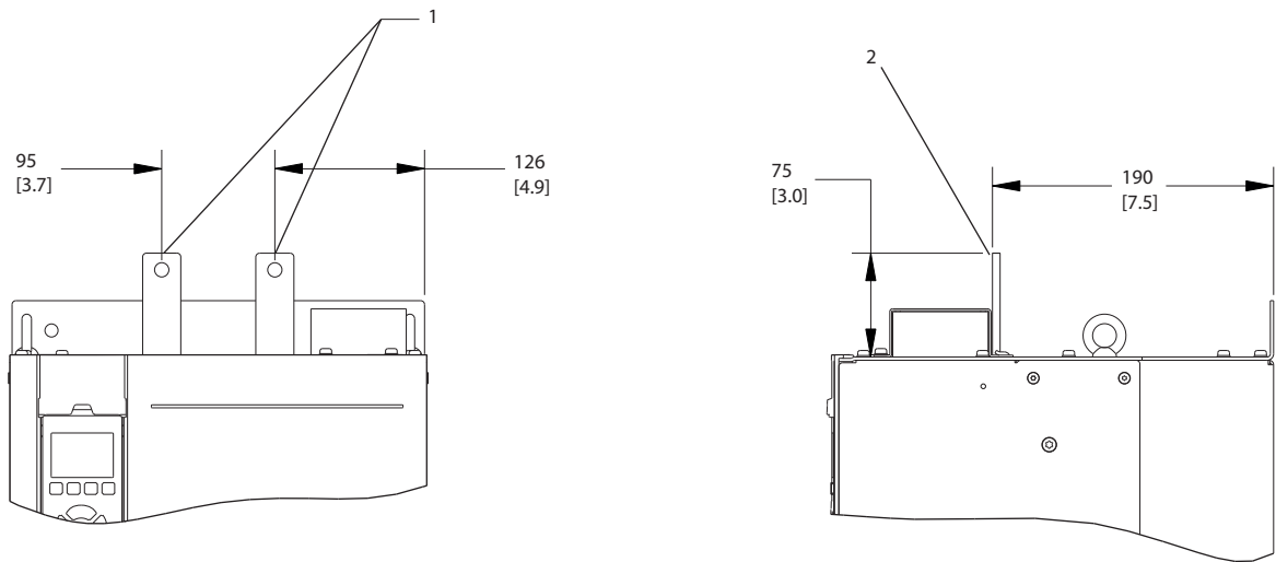
Εικόνα 2.12 Ακροδέκτες διαμοιρασμού φορτίου και αναδημιουργίας, D4h
