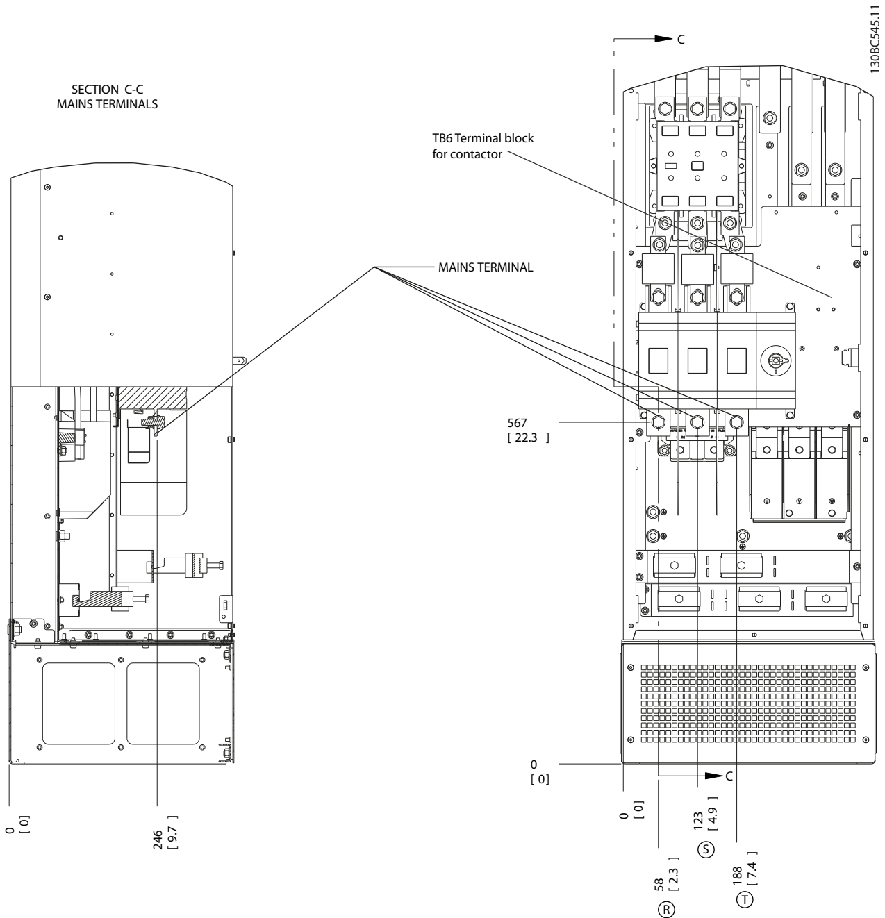
Εικόνα 2.21 Θέσεις ακροδεκτών, D8h με επιλογές Επαφές και Αποζεύκτη
