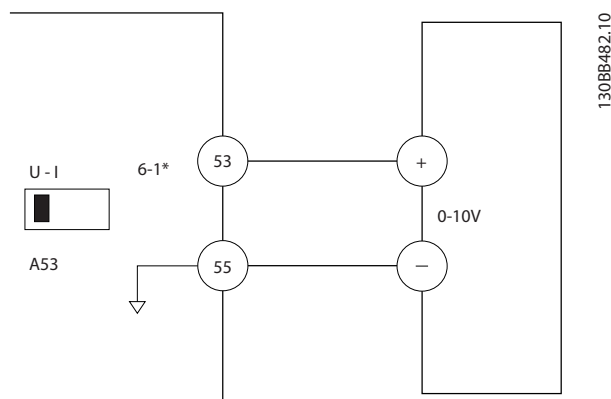
Ilustracija 5.10 Primer ožičenja za zunanjo napravo, ki dovaja 0–10 V krmilni signal
