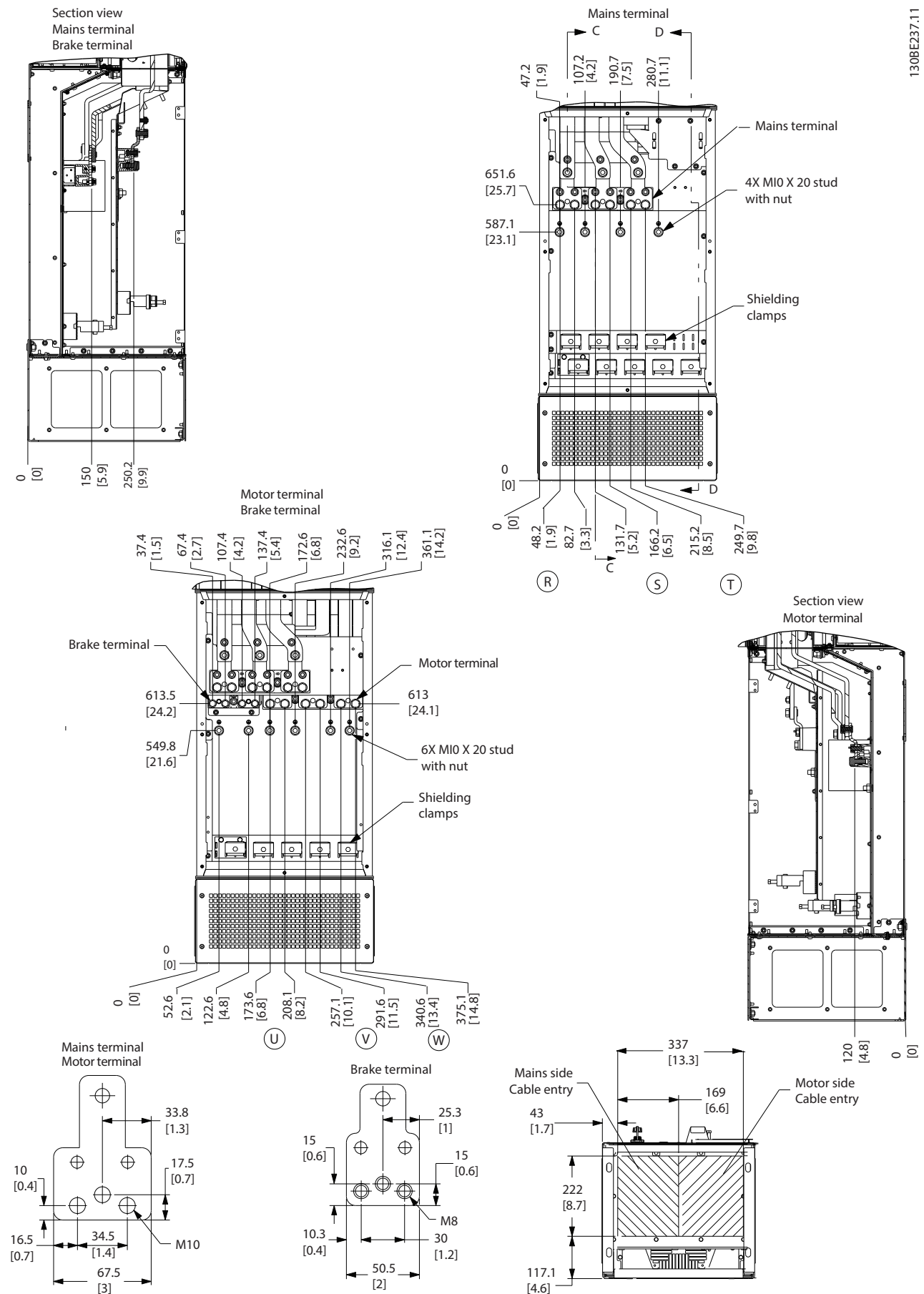
그림 4.19 대용량 배선 캐비닛, D7h
