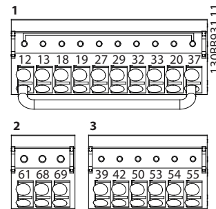
그림 4.25 단자 번호
