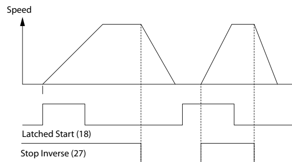
그림 6.3 펄스 기동/정지 인버스
