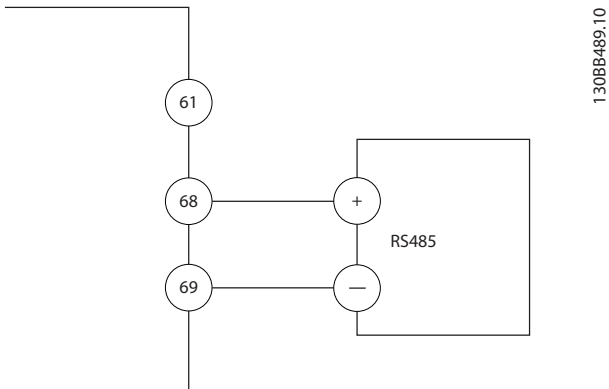
그림 4.28 직렬 통신 배선 다이어그램
