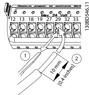
그림 4.26 제어 와이어 연결
