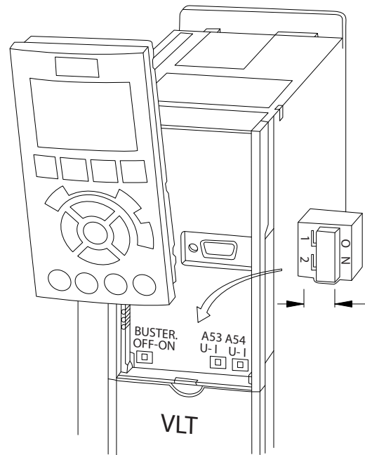
그림 4.27 단자 53 및 54 스위치의 위치
