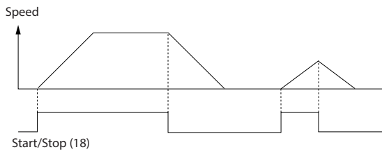
그림 6.2 STO가 있는 기동/정지 명령
