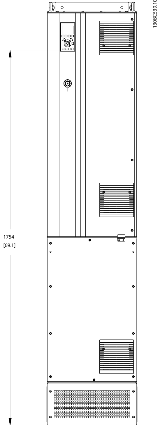
그림 1.2 D7h 외함
