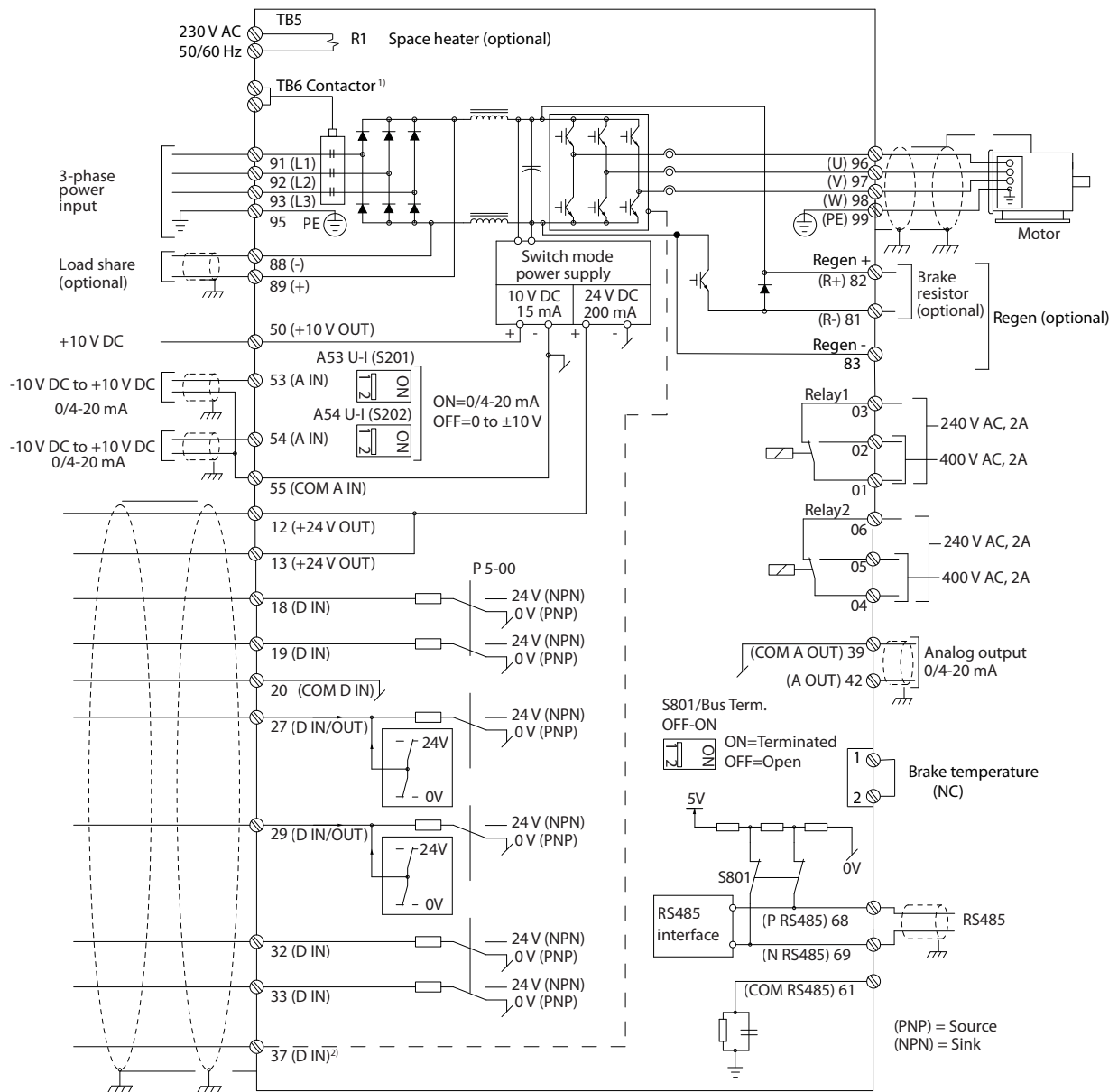
Illustration 5.2 Grundlæggende ledningsdiagram
