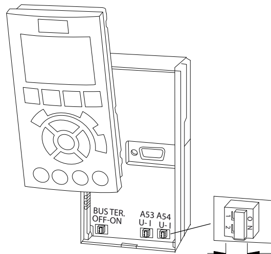
Illustration 5.40 Emplacement des commutateurs des bornes 53 et 54
