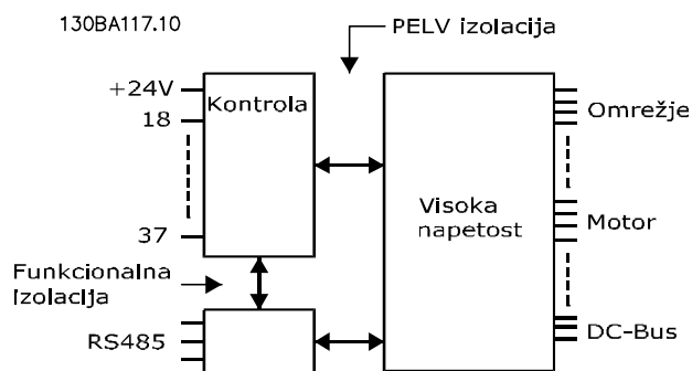
Ilustracija 10.1 Izolacija PELV
