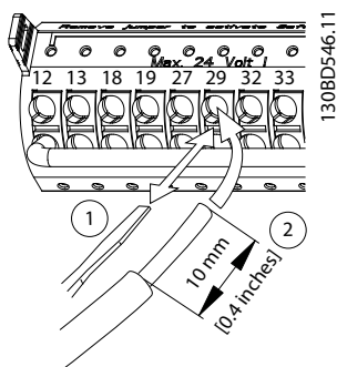
Ilustracija 5.38 Povezava upogljivih krmilnih kablov
