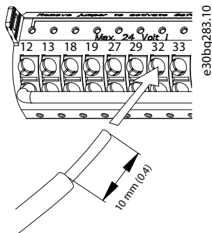
Ilustracija 5.37 Povezava trdnih krmilnih kablov
