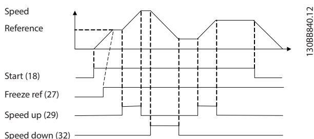
Slika 8.3 Ubrzanje/usporenje
