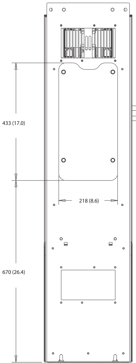
Slika 10.21 Dimenzije pristupa rashladnog tijela za D5h
