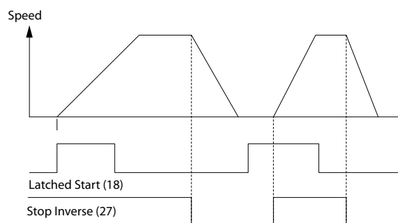
図 8.2 ラッチ・スタート/逆停止
