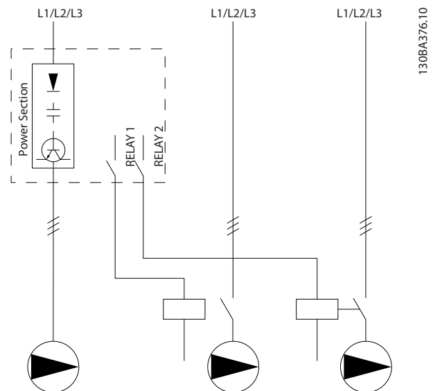
圖 8.5 固定/變動轉速泵浦的線路圖
