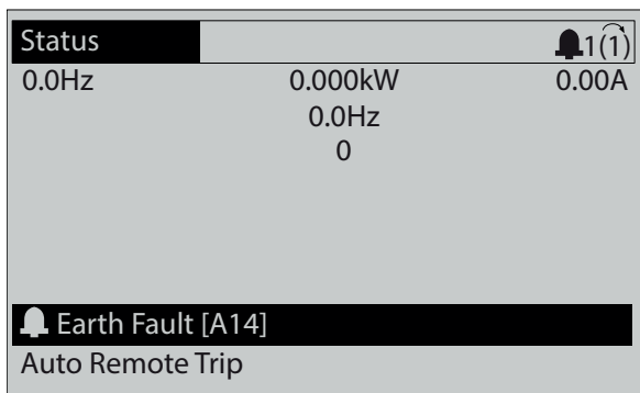
Ilustracja 9.3 Przykład alarmu
