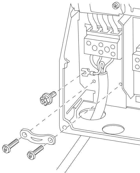
Рисунок 2.25 Подключение к сети и заземление, корпуса В1 и В2
