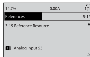
Рисунок 5.1 Пример программирования, шаг 1
