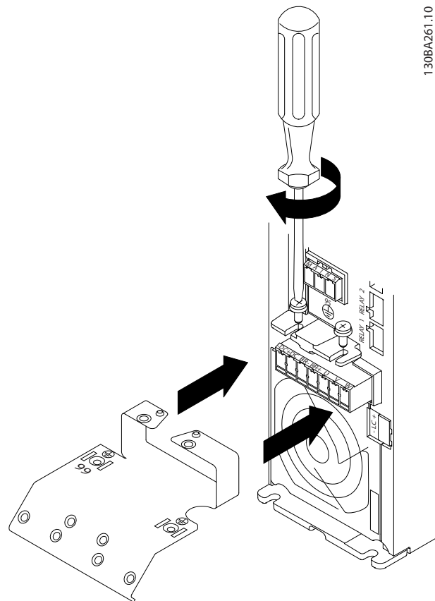
Рисунок 2.19 Положение монтажной платы
