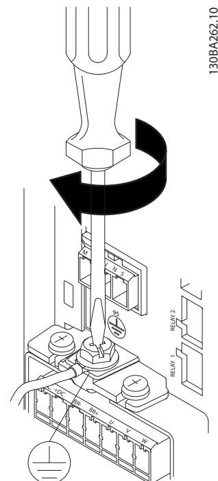
Рисунок 2.20 Монтаж кабеля заземления
