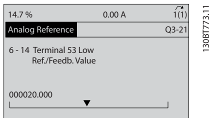
Рисунок 5.6 Пример программирования, шаг 6
