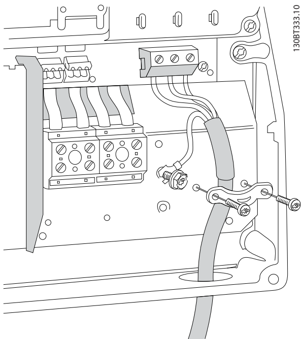
Рисунок 2.16 Подключение двигателя, корпуса В1 и В2
