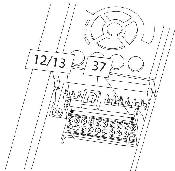
Рисунок 2.35 Перемычка между клеммой 12/13 (24 В) и клеммой 37
