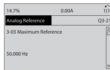
Рисунок 5.3 Пример программирования, шаг 3
