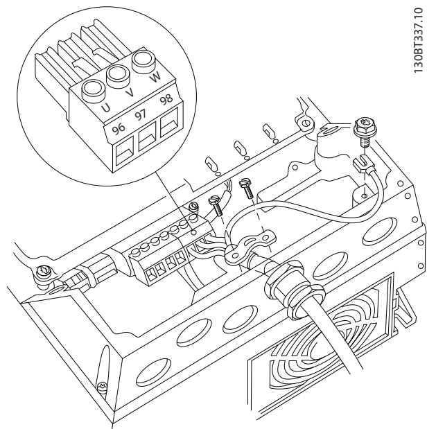
Рисунок 2.15 Подключение двигателя, корпуса A4 и A5
