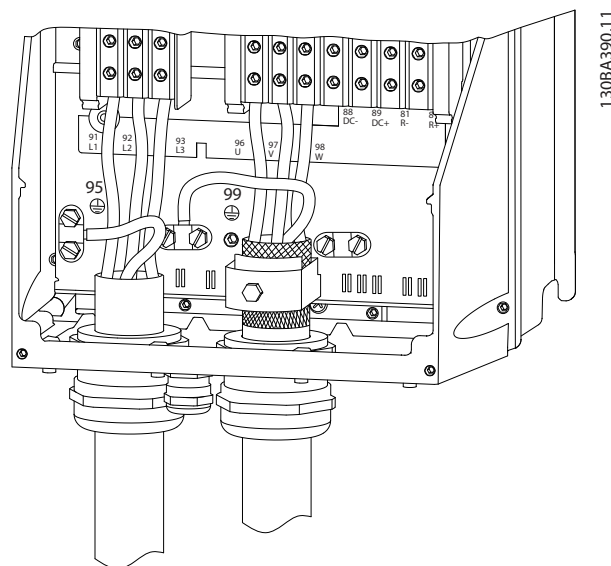
Рисунок 2.17 Подключение двигателя, корпуса С1 и С2
