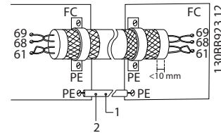
Рисунок 2.32 Кабели из витой пары
