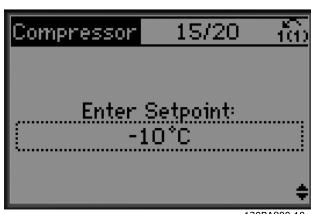
Рисунок 3.17 Задание уставки
