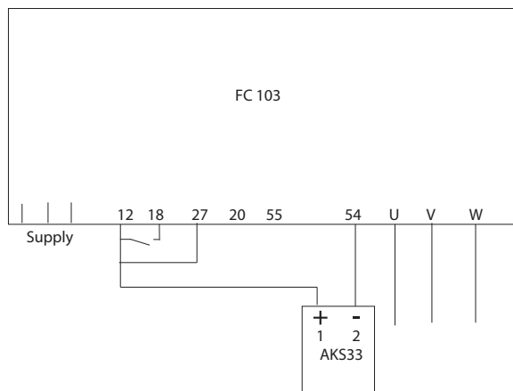
Рисунок 6.5 Как подсоединить FC 103 и AKS33 для применения с замкнутым контуром
