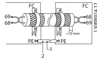
Рисунок 2.33 Кабели из витой пары без клеммы 61
