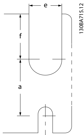
Ilustrația 3.5 Orificii de fixare în partea de sus și în partea de jos (B4, C3, C4)
