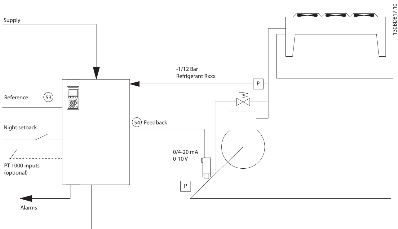
Ábra 6.1 A „belső vezérlésű kompresszor” standard rajza
