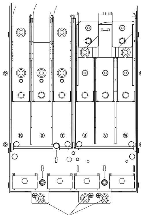
图 2.5 IP20（机架式）机箱的接地点
