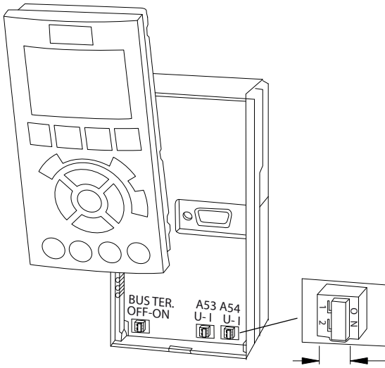
Çizim 5.22 Terminal 53 ve 54 Anahtarlarının Yeri
