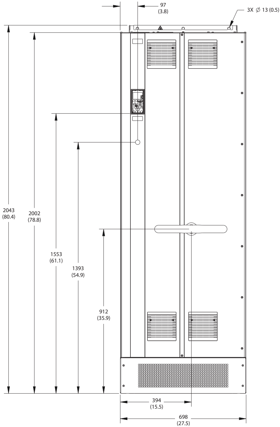
Çizim 9.6 E2h'nin Önden Görünümü
