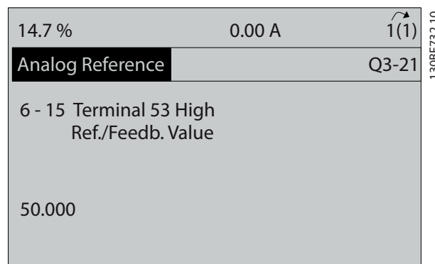
Illustration 6.11 Paramètre 6-15 Val.ret./Réf.haut.born.53
