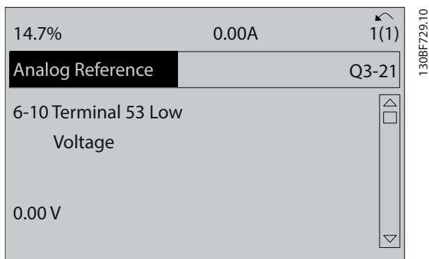
Illustration 6.8 Paramètre 6-10 Ech.min.U/born.53
