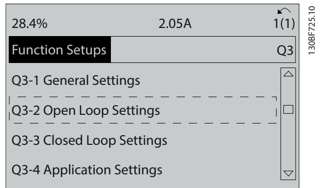
圖 6.4 Q3-2 開迴路設定
