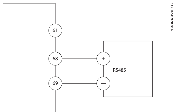
圖 5.21 串列通訊配線圖
