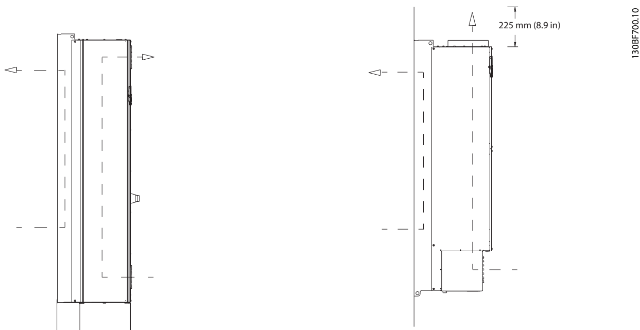
Afbeelding 9.19 Luchtstroom bij gebruik van backchannelkoelsets op E1h/E2h (links) en E3h/E4h (rechts)
