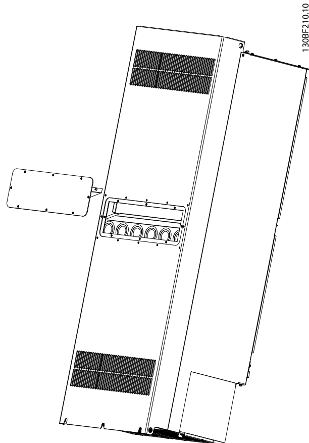
Abbeelding 8.1 Toegangspaneel koellichaam verwijderd van de achterzijde van de frequentieregelaar
