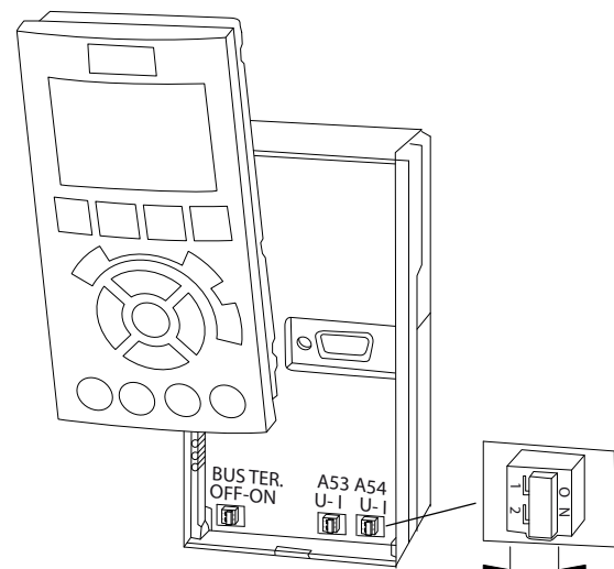
圖 5.22 端子 53 和 54 開關的位置
