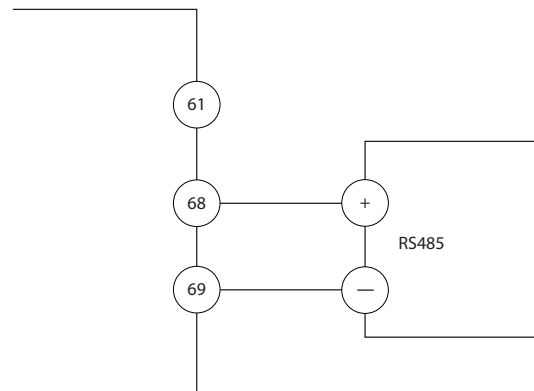
圖 5.21 串列通訊配線圖
