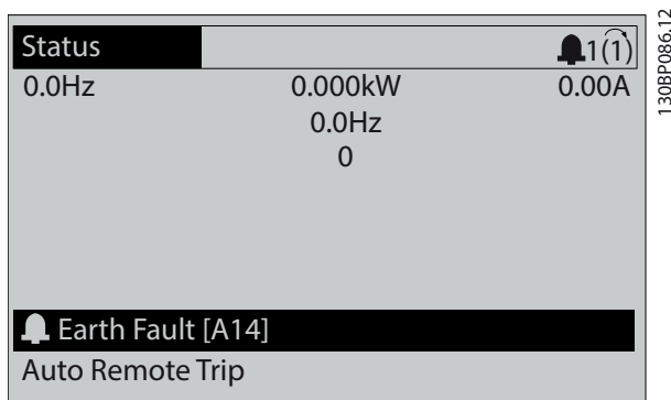
圖 8.3 警報範例
