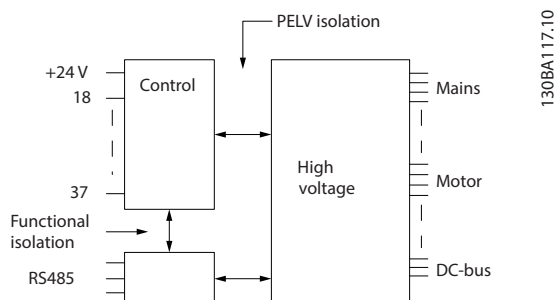
圖 9.1 PELV 絕緣
