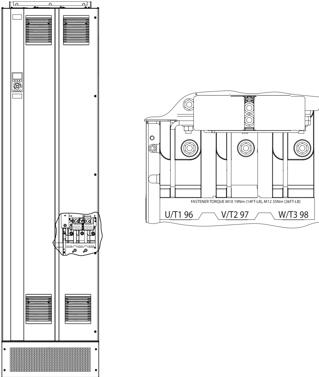
圖 5.3 AC 馬達端子 (如 E1h 所示)。如需端子的詳細檢視，請參考 章 5.7 端子尺寸
