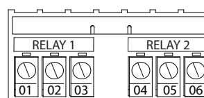
Slika 5.19 Priklučki releja 1 i releja 2
