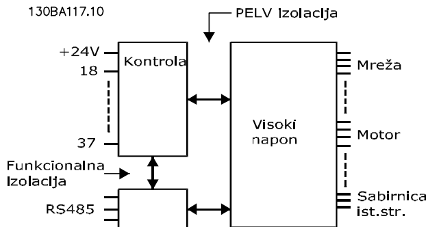
Slika 9.1 PELV izolacija
