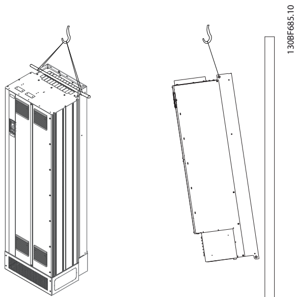
Ilustrația 4.2 Metodă de ridicare recomandată
