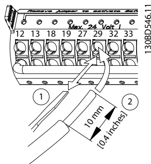
Ilustrația 5.20 Conectarea cablurilor de control
