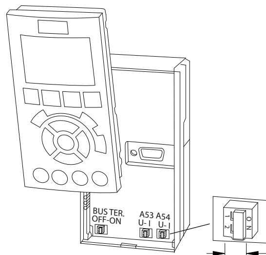
Illustration 5.23 Placering af kontakter til klemme 53 og 54
