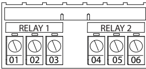
Slika 5.19 Stezaljke releja 1 i releja 2
