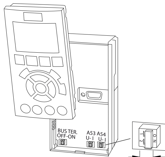
Slika 5.23 Lokacija sklopki stezaljki 53 i 54
