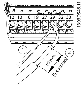
Slika 5.21 Spajanje fleksibilnih upravljačkih žica
