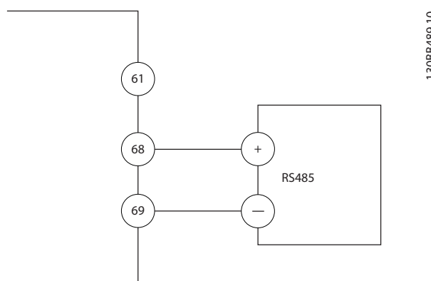
Slika 5.22 Shema spajanja serijske komunikacije
