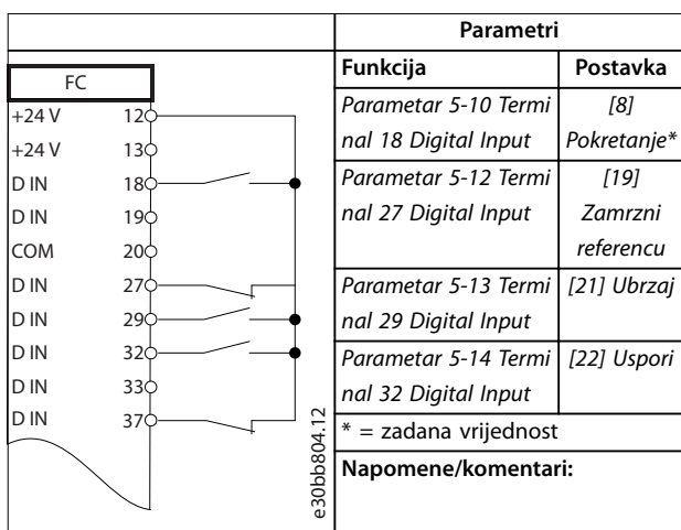
Tablica 7.4 Ubrzanje/usporenje
