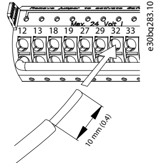
Slika 5.20 Spajanje čvrstih upravljačkih žica
