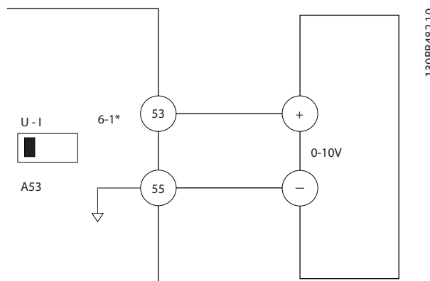
Slika 6.12 Primjer ožičenja za vanjski uređaj koji daje upravljački signal 0 – 10 V
