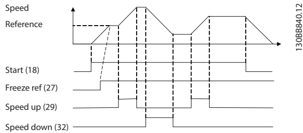
図 7.1 加速/減速
