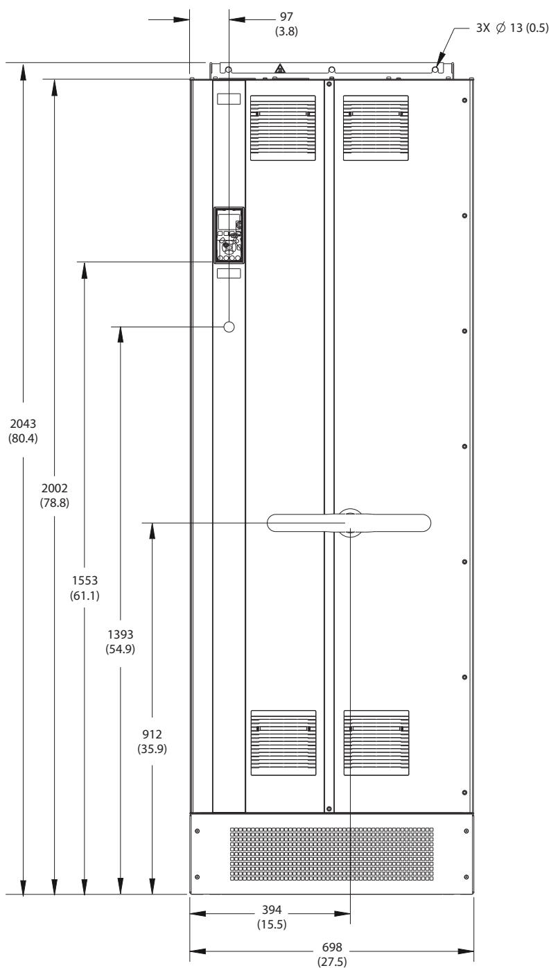
圖 9.6 E2h 的正面圖
