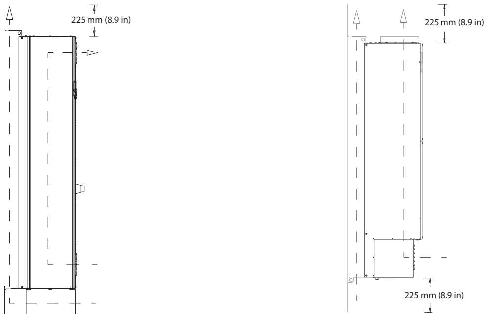
圖 9.18 E1h/E2h (左) 與 E3h/E4h (右) 的標準空氣氣流配置
