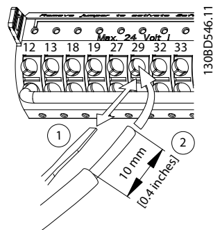
Slika 5.21 Priključivanje fleksibilnih upravljačkih provodnika
