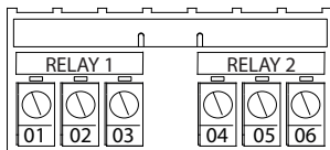
Slika 5.19 Priključci releja 1 i releja 2
