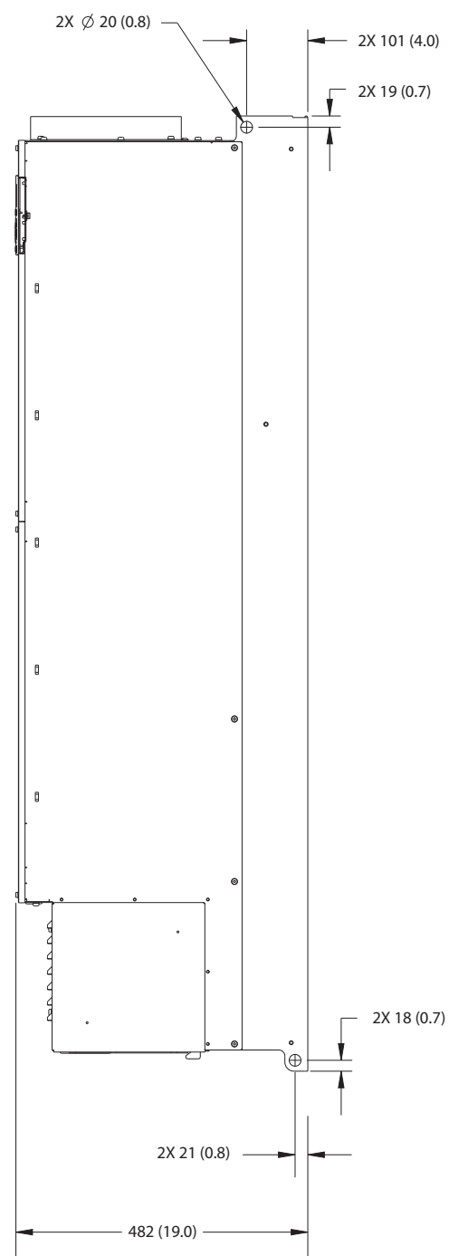
Ábra 9.15 Az E4h oldalnézete
