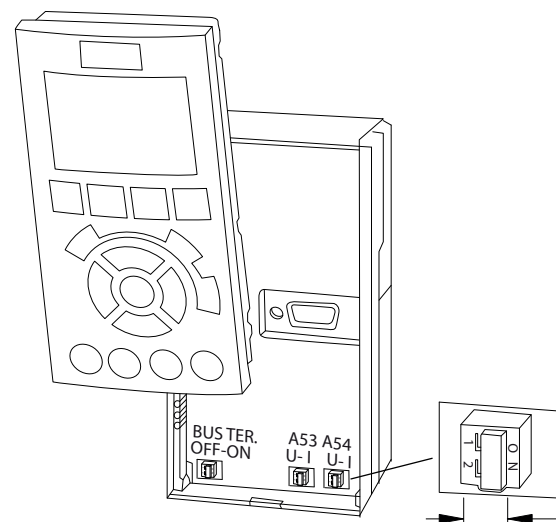
Ábra 5.23 Az 53-as és az 54-es csatlakozó kapcsolójának elhelyezkedése
