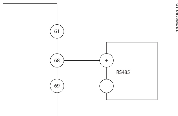
Ábra 5.22 A soros kommunikáció kapcsolási rajza
