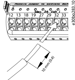
Ilustrasi 5.20 Menghubungkan Kabel Kontrol Solid
