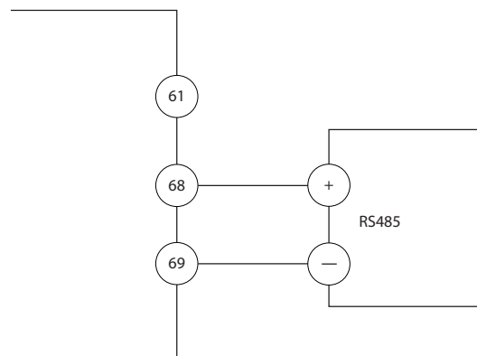
Ilustrasi 5.22 Diagram Kabel Komunikasi Serial
