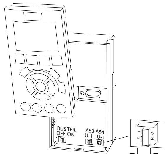
Ilustrasi 5.23 Lokasi Saklar Terminal 53 dan 54
