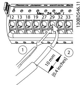
Ilustrasi 5.21 Menghubungkan Kabel Kontrol Fleksibel
