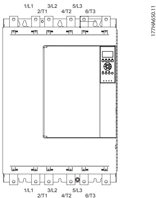
Ilustração 4.6 MCD5-0469B a MCD5-0961B, 469-961 A
