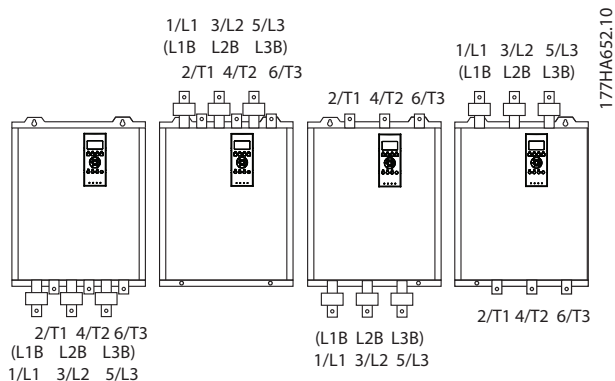
Ilustração 4.8 Localização dos terminais de bypass, MCD5-0360C para MCD5-1600C, 360-1600 A
