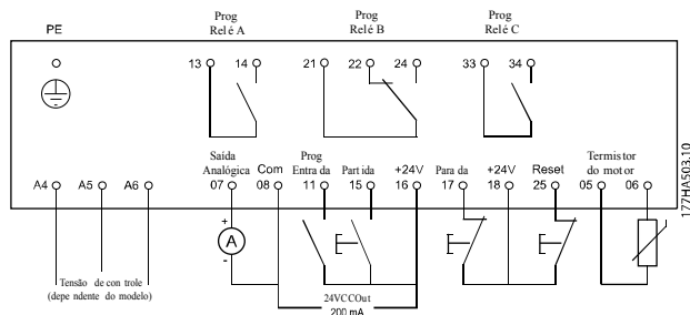
Ilustração 4.1 Fiação para os Terminais de Controle
