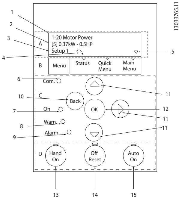
Abbildung 1.27 Bedieneinheit (LCP)
