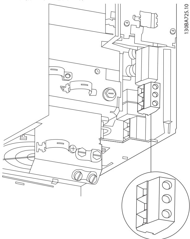
图 3.12 H10 机箱
