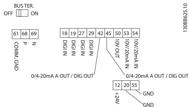
图 3.23 控制端子
