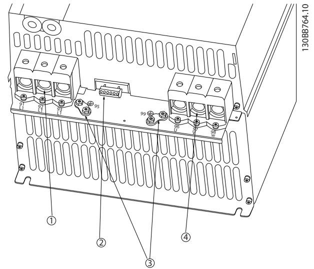
H8 机箱上的继电器和端子
