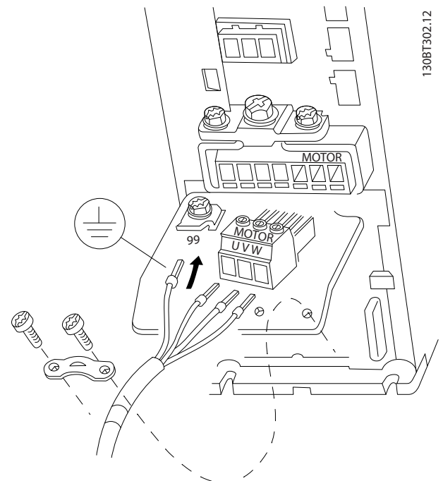
图 3.7 将变频器连接到电机, H9 机箱
