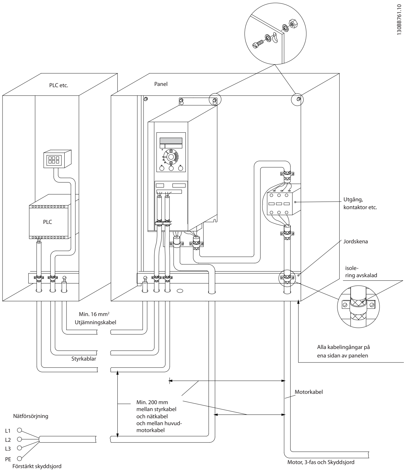
Bild 3.21 EMC-korrekt installation
