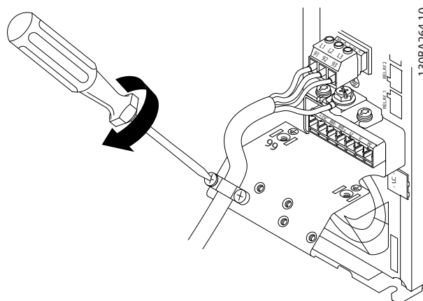
Slika 3.11 Ugradnja potpornog elementa
