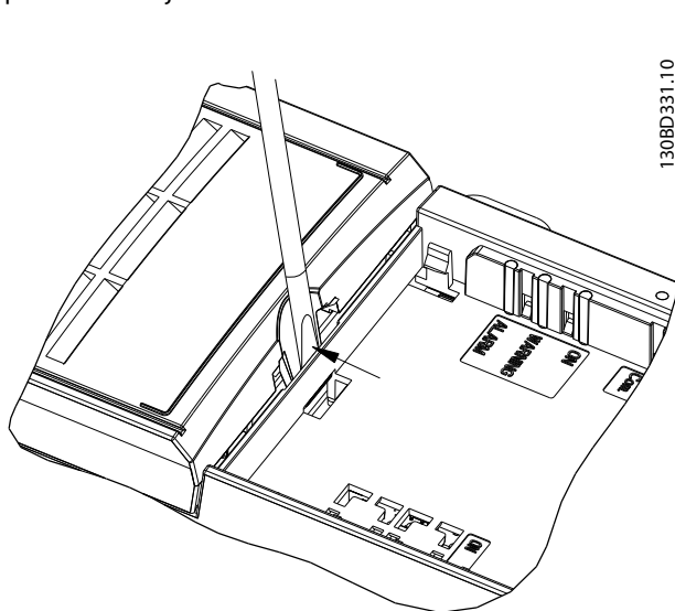
Slika 3.22 Uklanjanje pokrova stezaljke
