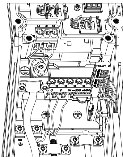
圖 3.16 IP54 外殼規格 I2、I3、I4
