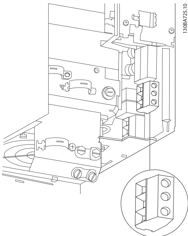
圖 3.12 外殼規格 H10
