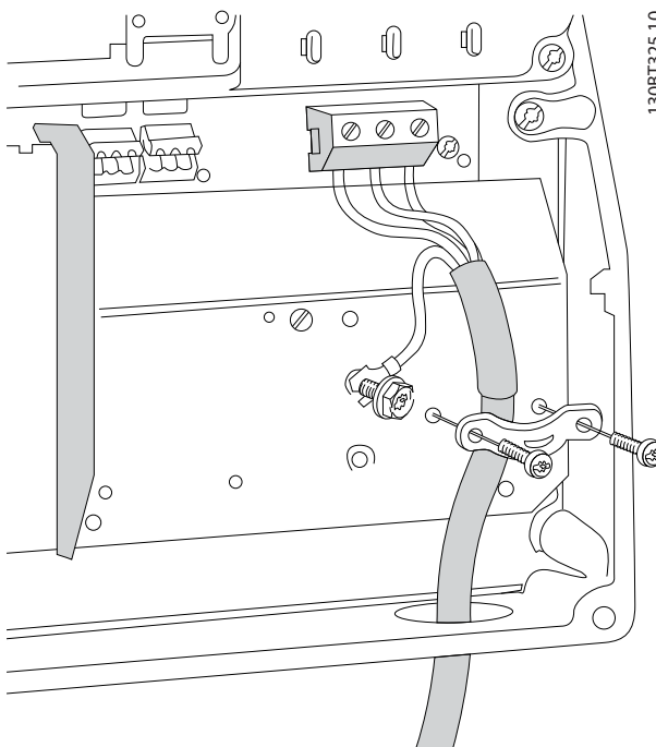
Εικόνα 3.18 Σύνδεση στον κινητήρα για το Μέγεθος περιβλήματος Ι6 IP54, 380–480 V, 22–37 kW (30–50 hp)
