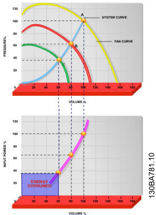
Рисунок 2.2 Если использовать преобразователи частоты для снижения мощности вентиляторов до 60 %, в типовых условиях применения можно сэкономить до 50 % электроэнергии.
