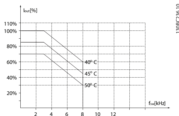
Рисунок 8.20 600 В, IP20, H8, 75–90 кВт
