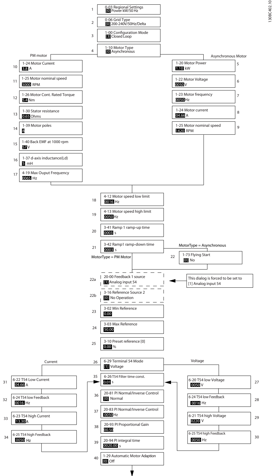
Рисунок 2.22 Мастер настройки параметров замкнутого контура
