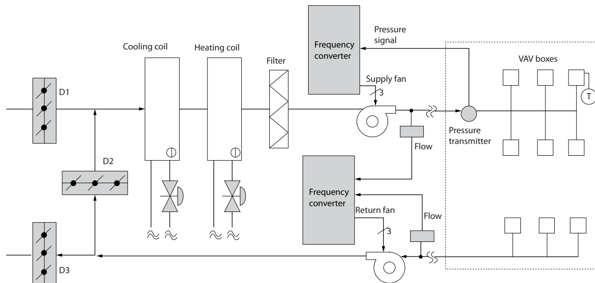
Рисунок 2.11 Переменный объем воздуха
