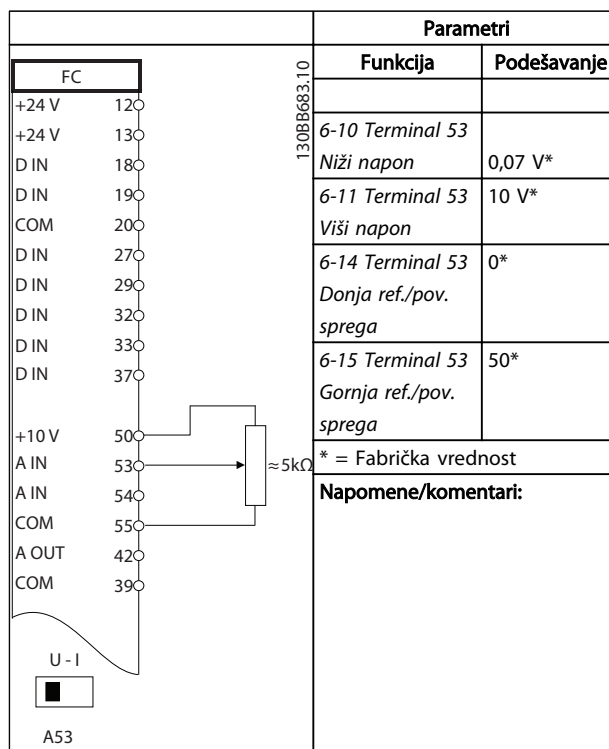
Tablica 6.9 Referenca brzine (pomoću ručnog potencijometra)
