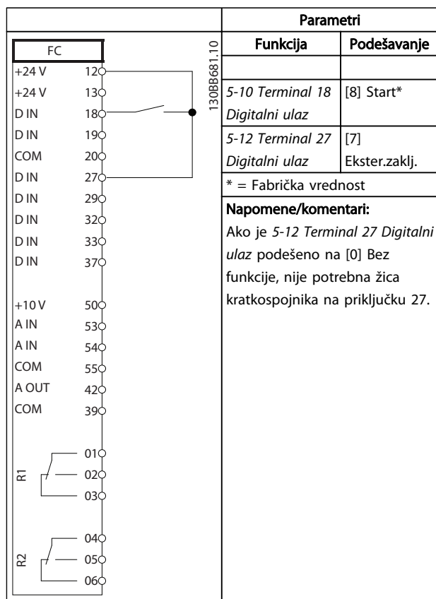
Tablica 6.7 Komanda za pokretanje/zaustavljanje bez eksterne blokade rada
