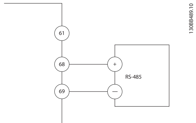
Slika 2.22 Dijagram ožičenja serijske komunikacije
