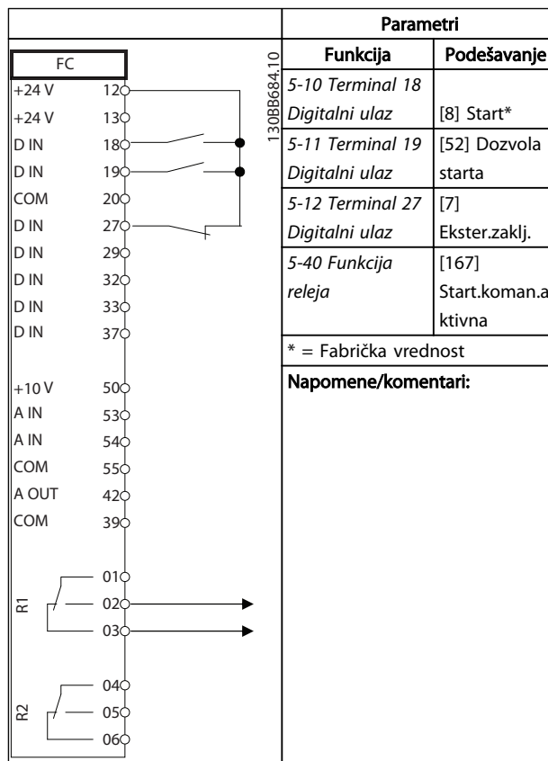
Tablica 6.10 Dozvola starta
