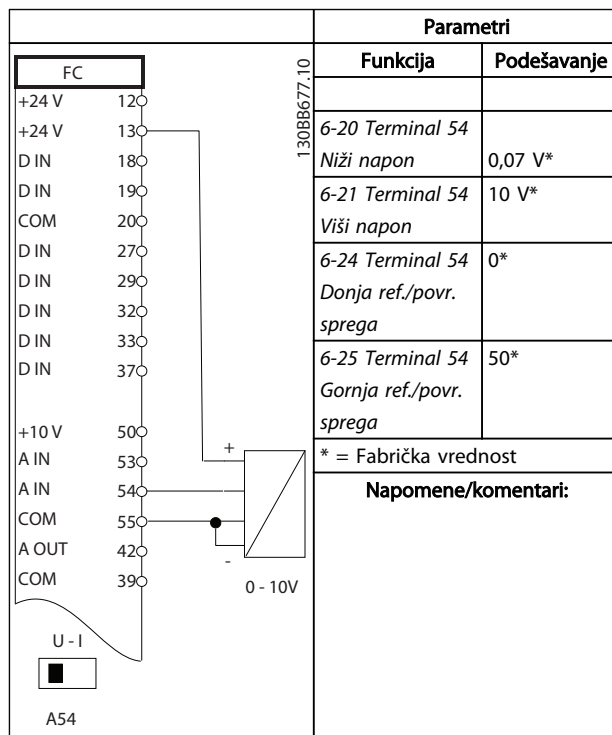
Tablica 6.3 Analogni naponski pretvarač signala povratne sprega (4-žični)
