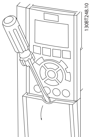
Slika 2.12 Pristup ožičenju upravljanja za kućišta A2, A3, B3, B4, C3 i C4
