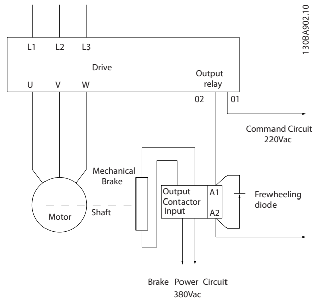
Slika 2.21 Prikjučivanje mehaničke kočnice na frekventni pretvarač
