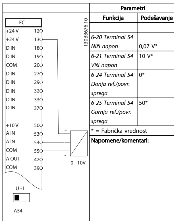
Tablica 6.2 Analogni naponski pretvarač povratne sprega (3-žični)
