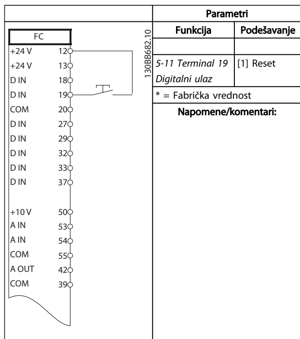
Tablica 6.8 Eksterni reset alarma
