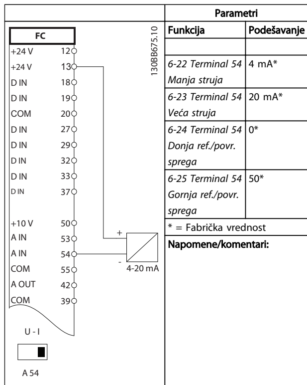
Tablica 6.1 Analogni strujni pretvarač povratne sprega
