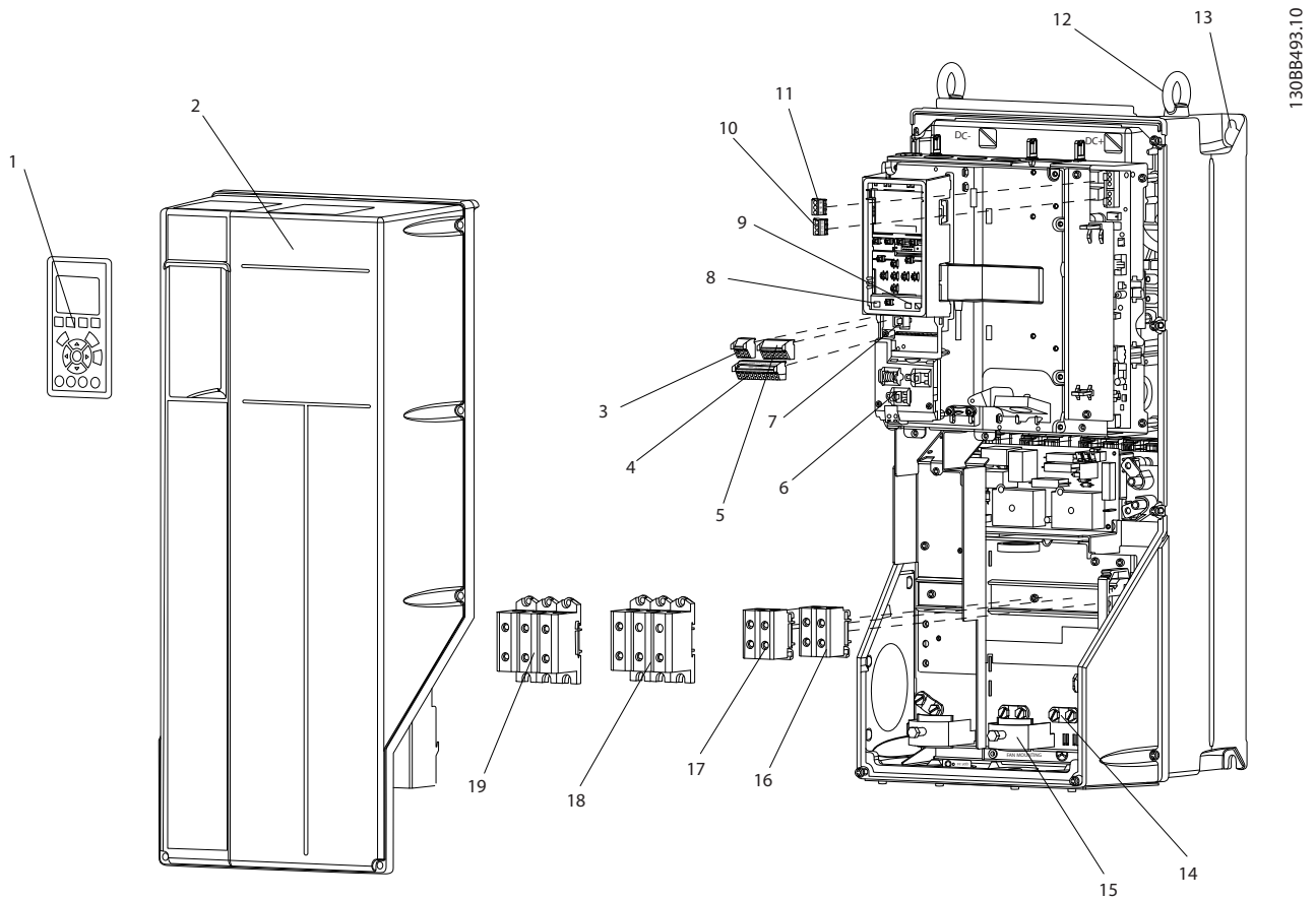
Рисунок 1.2 Раздельный обзор, вид В и С
