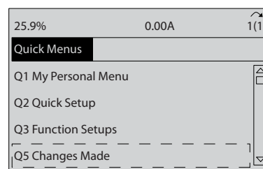
Рисунок 5.12 Быстрые меню
