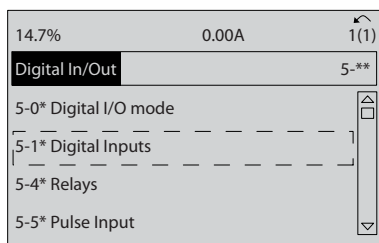
Рисунок 5.10 Цифр. вход/выход
