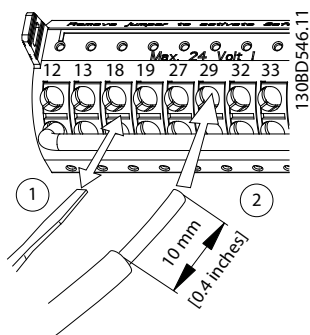
Kuva 4.9 Ohjauskaapeleiden kytkentä
