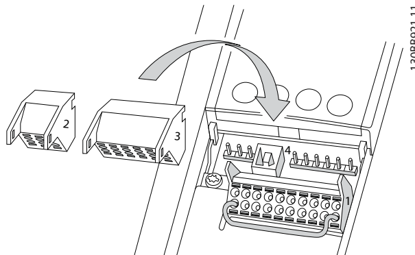
Kuva 4.7 Ohjusliitinten paikat
